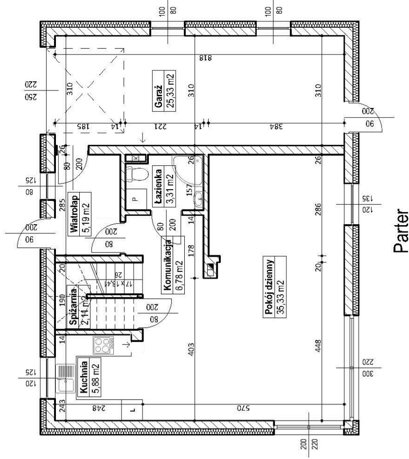
ZESTAWIENIE POWIERZCHNI PARTERU DLA LOKALU MIESZKALNEGO:
