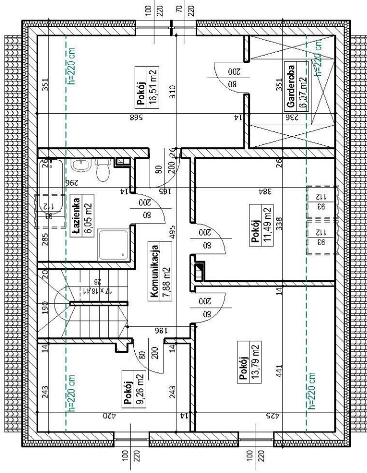
ZESTAWIENIE POWIERZCHNI PIĘTRA DLA LOKALU MIESZKALNEGO:
